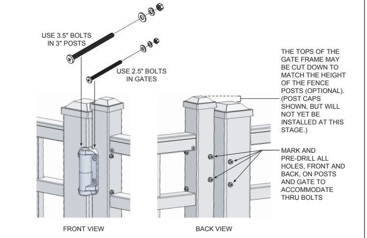
Dia. 7
