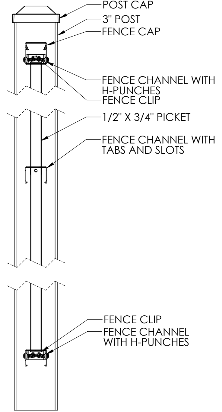
SECTION A-A
